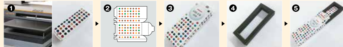
1 Impression directe sur clé USB 2 Impression sur carton compact couché 3 Découpe du carton imprimé pour réaliser l'emballage 4 Découpe du matériau de calage 5 Assemblage des différentes parties pour le façonnage !
